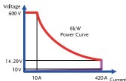
PEL-5006C-600-420
