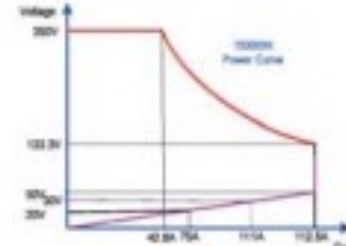
AEL-5015-350-112.5
