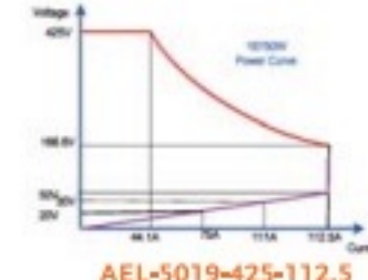
AEL-5019-425-112.5
