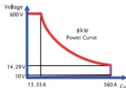
PEL-5008C-600-560
