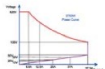
AEL-5004-425-37.5
