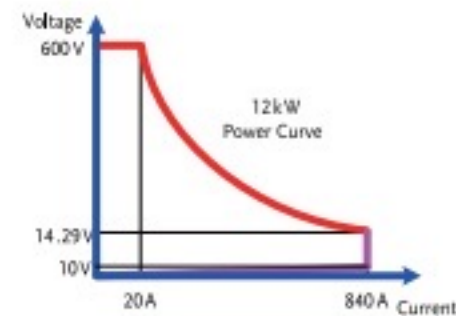
PEL-5012C-600-840
