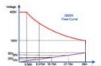
AEL-5003-425-28
