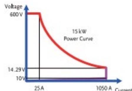
PEL-5015C-600-1050
