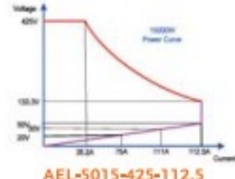
AEL-5015-425-112.5
