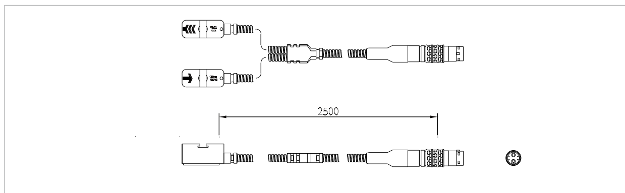
Transducteurs K4N/E
