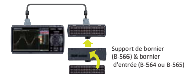
Bornier d'entrée (B-564/565)
