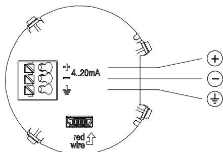
Cable gland
